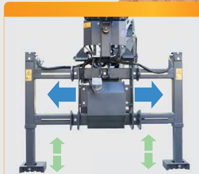
Pies de apoyos independientes con valulas de bloque. Posibilidad de aumentar la traslación para permitir el trabajo en cualquier condición y en toda seguridad.
